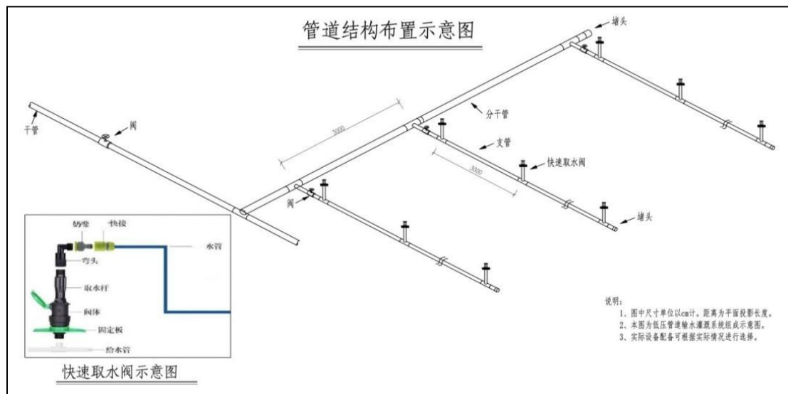
图 7-2 水肥一体化灌溉系统管道架构布置示意图
