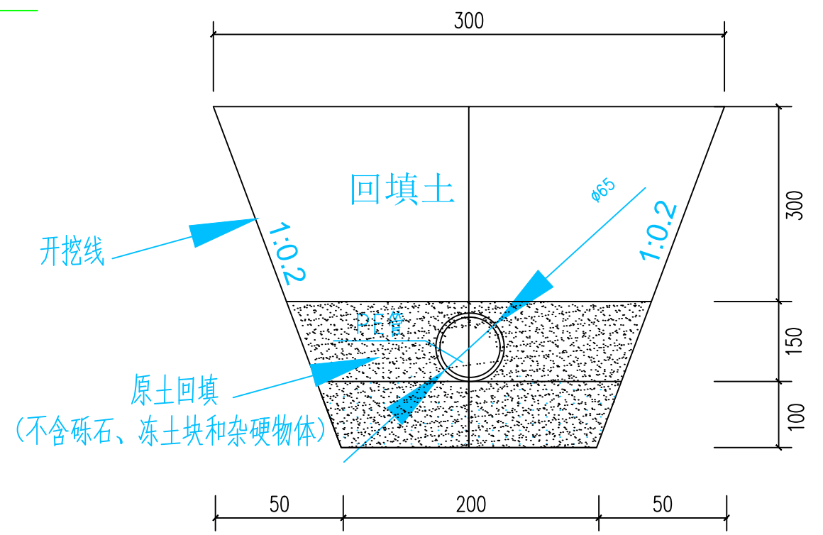
沿山管道开挖断面图
