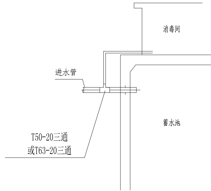
消毒器进水示意图
