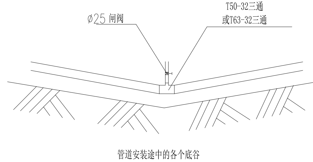
高处排气阀示意图
