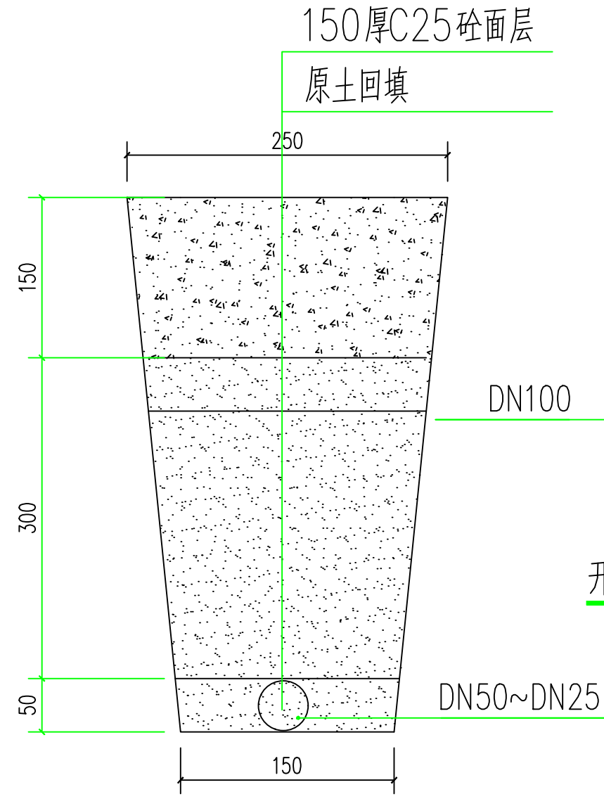
② 开挖村内砼路面恢复大样 1:5
